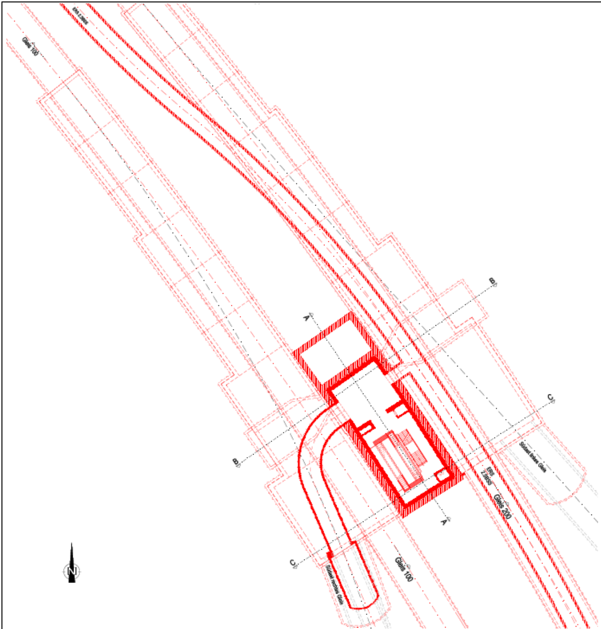
Bild 24: Rettungsschacht Nr. 7 mit Fahrtreppen und Festtreppe (Grundriss Ebene -5 mit Anschlüssen der Erkundungs- und Rettungsstollen der 2. SBSS und des Südabzweigs, Prinzip)
