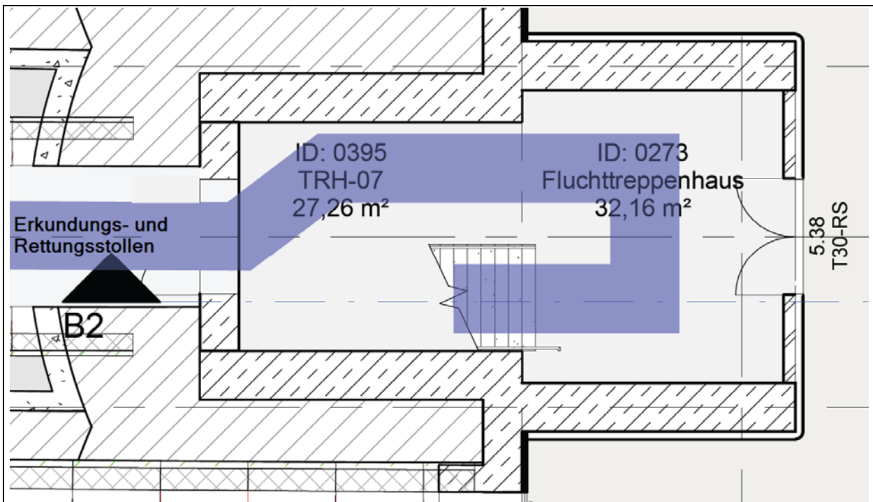
Bild 17: Anschluss des Erkundungs- und Rettungsstollens an den Fluchttreppenraum Mitte am westlichen Bahnsteigende der uPva MMHO (Grundriss, Prinzip)
