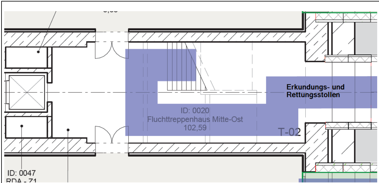
Bild 16: Anschluss des Erkundungs- und Rettungsstollens an den Fluchttreppenraum Mitte am östlichen Bahnsteigende der uPva MHP (Grundriss, Prinzip)
